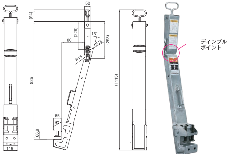
規格寸法
