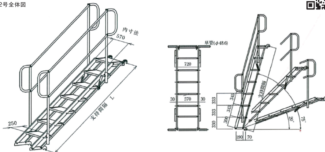
法面2号全体図
